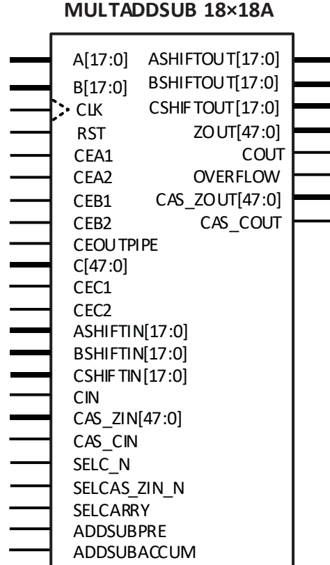
Figure 3.7. MULTADDSUB18×18A Primitive
