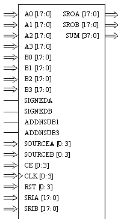
MULT18x18ADDSUBSUMB
