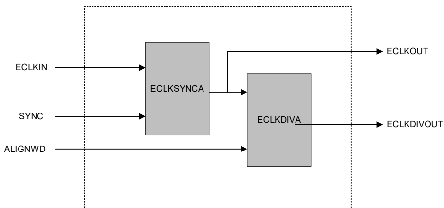
Figure 2.10. ECLKSYNCDIV
