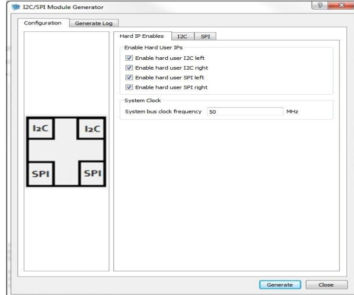
Figure 3-25 : Enable Hard IP
