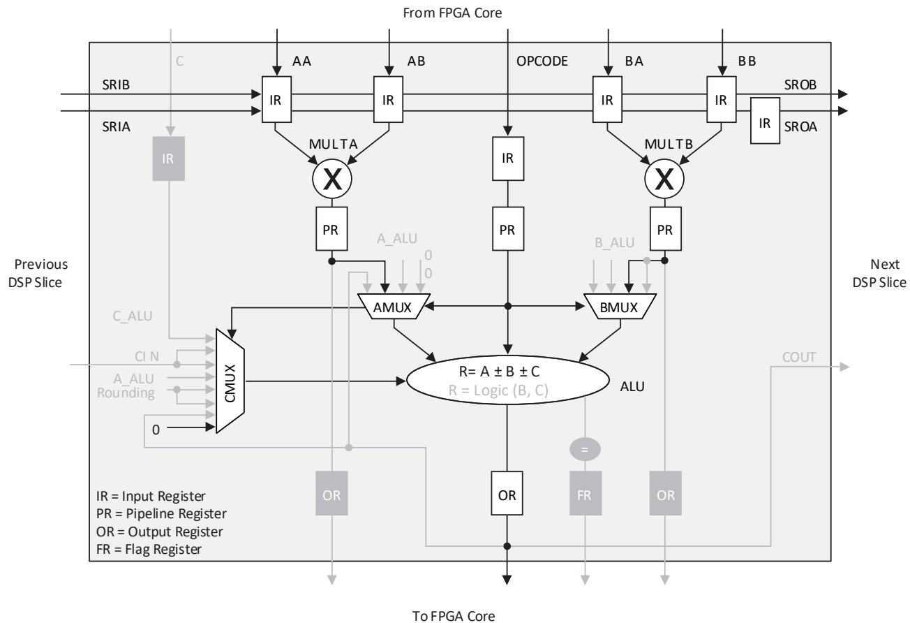
Figure 2.29. MULTADDSUB
