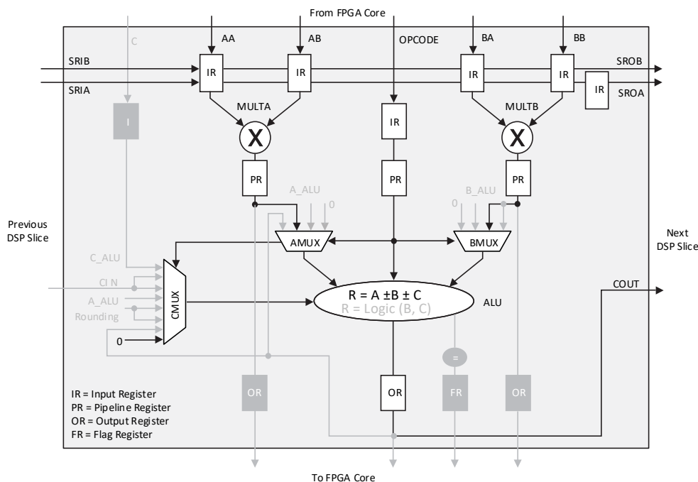
Figure 2.30. MULTADDSUBSUM Slice 0
