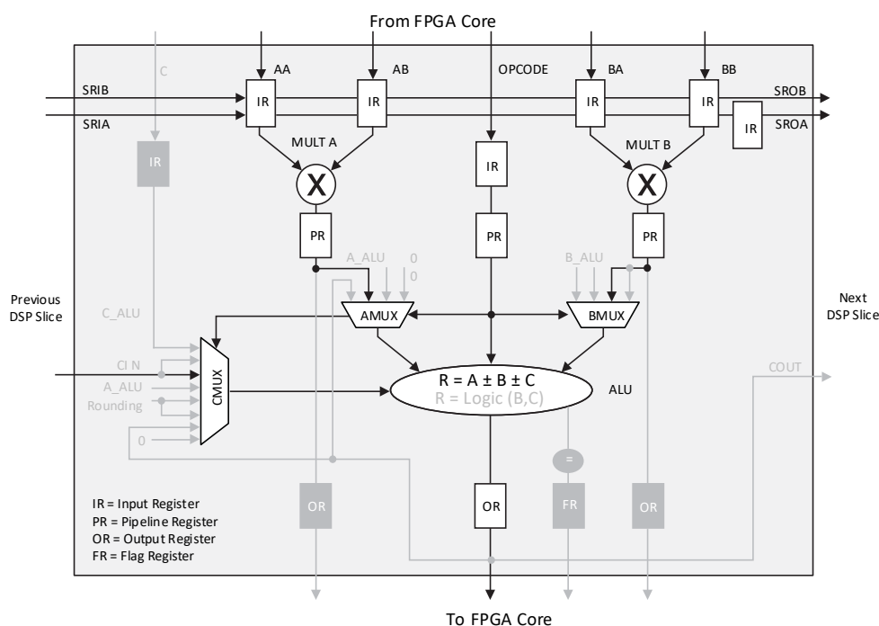
Figure 2.31. MULTADDSUBSUM Slice 1
