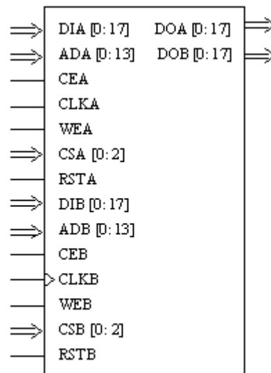
DP16KB
