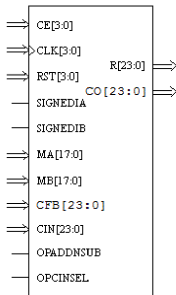
ALU24B
